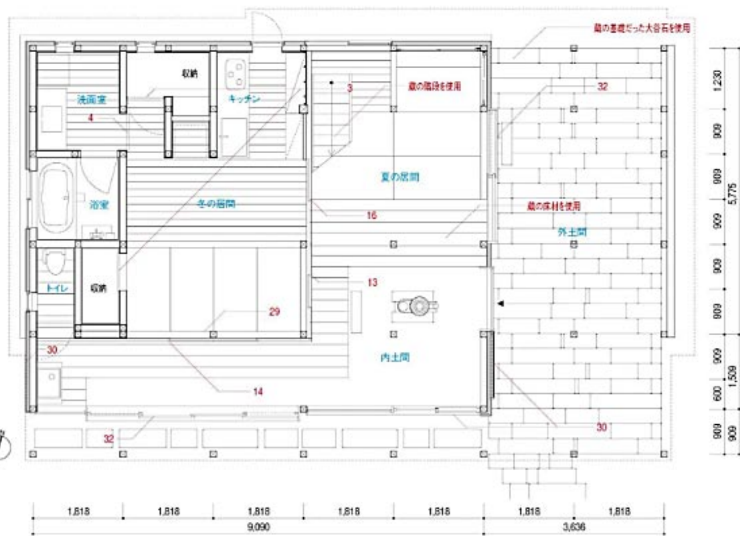
1階平面図
